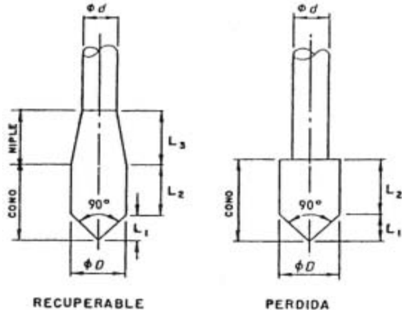
FIG. 9 - Alternativas de cono
