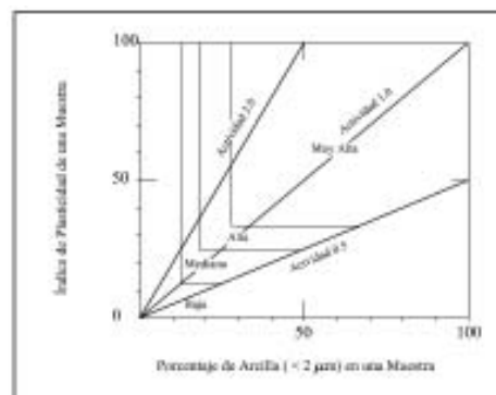
GRÁFICO 6.3.1 CLASIFICACIÓN DE CAMBIO DE POTENCIAL DE VOLUMEN PARA SUELOS ARCILLOSOS
