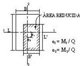
(B) ÁREA REDUCIDA - CIMIENTO RECTANGULAR
