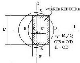
(C) ÁREA REDUCIDA - CIMIENTO CIRCULAR
