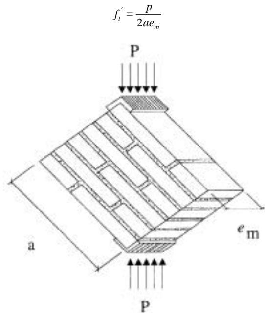
FIGURA 7 ENSAYO DE COMPRESIÓN DIAGONAL
