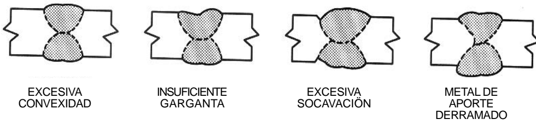
E) Perfiles de Soldadura Acanalada Inaceptables en Juntas a Tope
